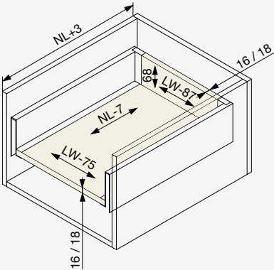
① Rozměry dna a zad zásuvky
